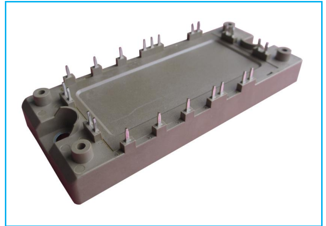
Rectifier+Brake+Inverter
